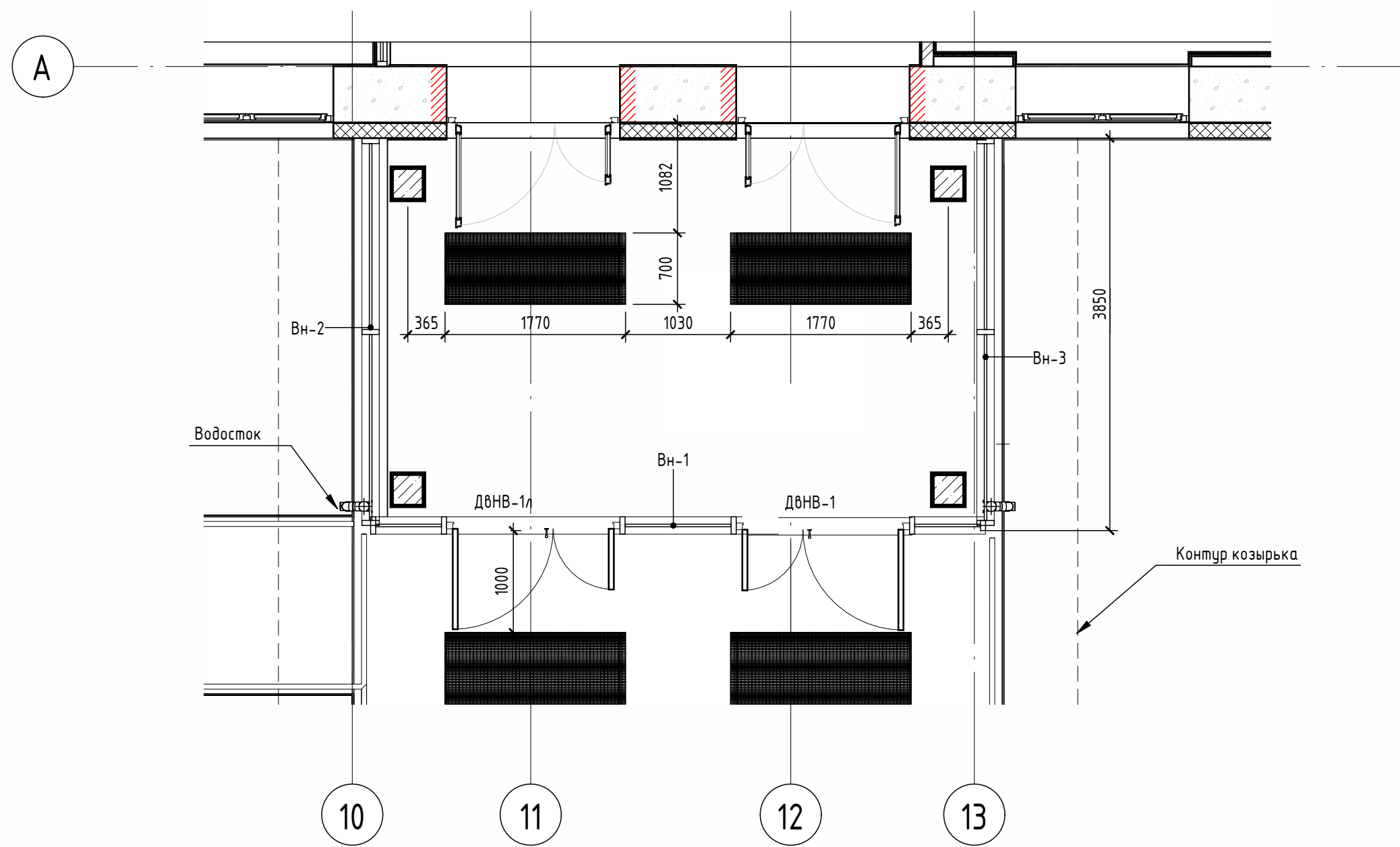
Фрагмент плана входной группы №1
