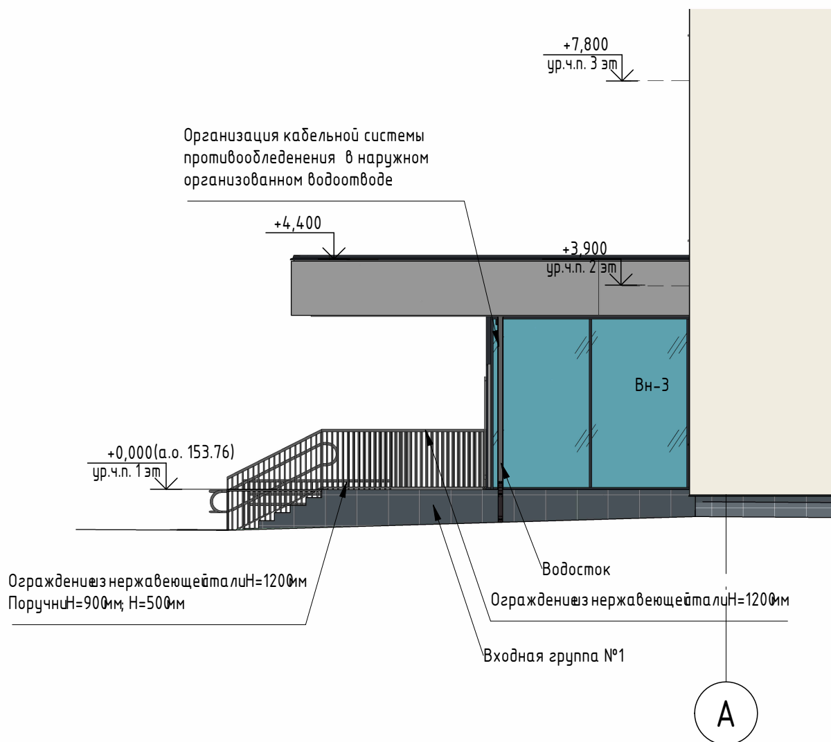
Фрагмент фасада в осях П-А
